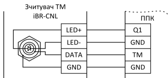
Рисунок 2.7 – Схема підключення зчитувача ключів ТМ
