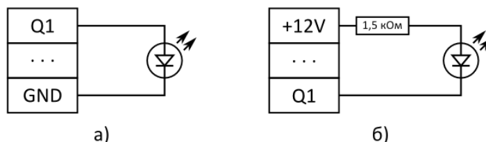
а) – до ППК або клавіатури (виносний світлодіод), в) – до ППК або клавіатури (відкритий колектор)
