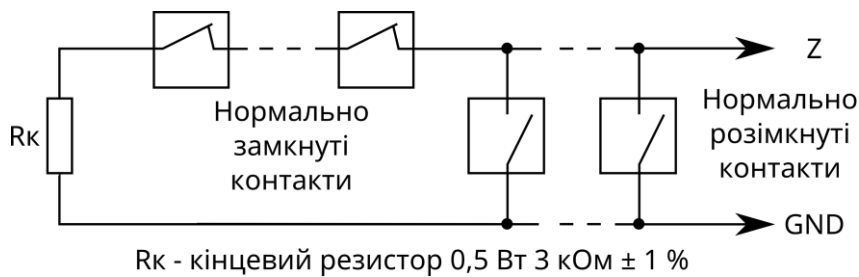
Рисунок 2.2 – Схема включення охоронних сповіщувачів з нормально замкнутими та нормально розімкнутими контактами
