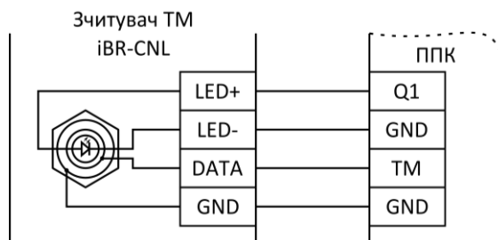
Рисунок 2.6 – Схема підключення зчитувача ключів ТМ
