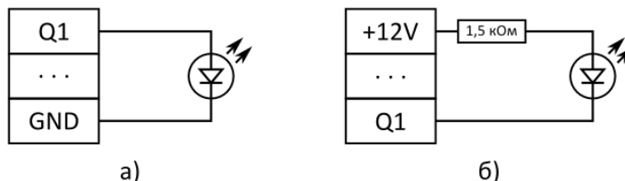
Рисунок 2.5 – Схеми підключення індикаторів підтвердження
