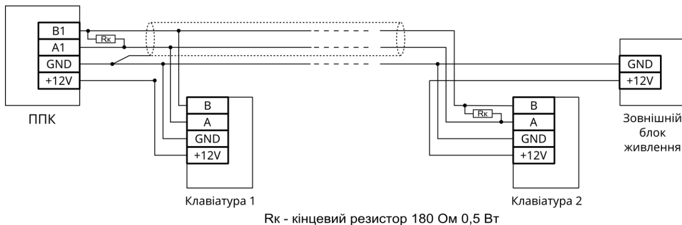
Рисунок 2.1 – Приклад підключення клавіатур по шині RS-485
