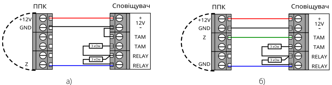
Рисунок 2.3 – Приклади підключення сповіщувачів по типу 2EOL
