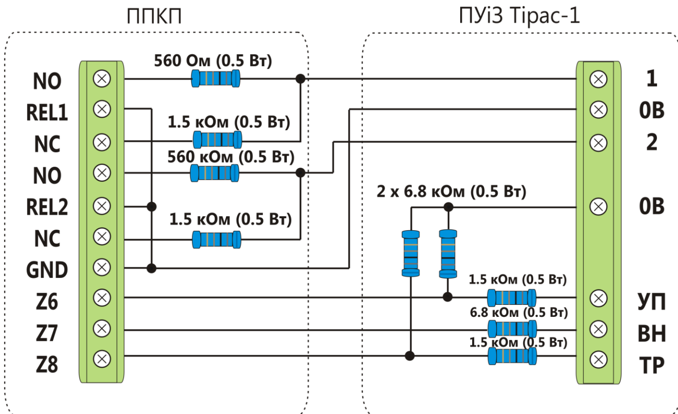
Рисунок 18 – Схема підключення ПУІЗ «Tiras-1».
